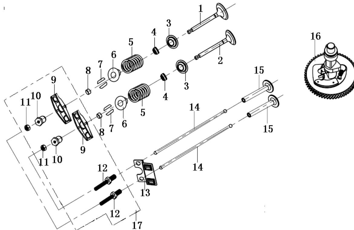
(Valve)
